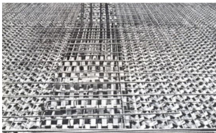
Esempio di solettone pronto per getto di calcestruzzo
